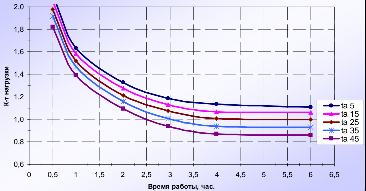
Нагрузочная характеристика ТСЗР-10
