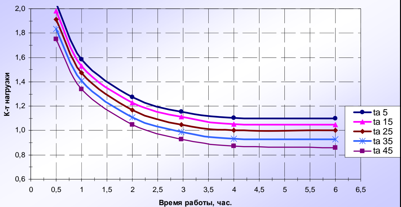
Нагрузочная характеристика ТСЗР-16
