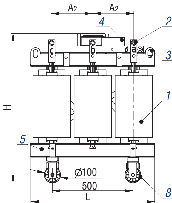
Вывод НН
