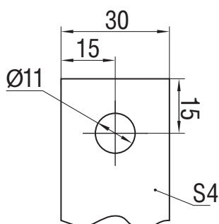
Вывод НН
